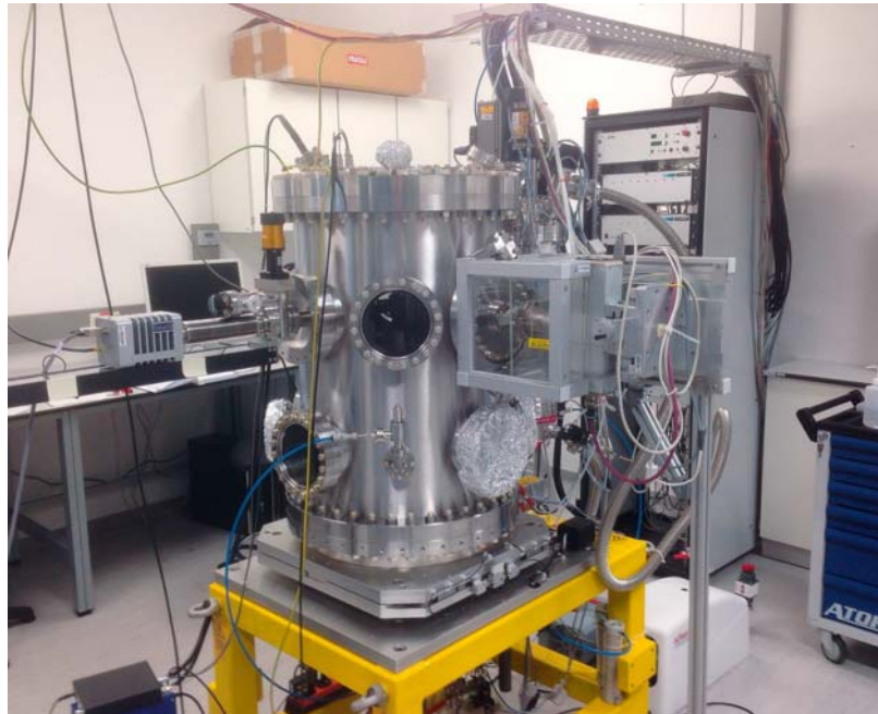
الشكل ٣ - سُنستخدم الحجرة الفانقة الفراغ في مختبر الوكالة في زايبيرسدورف لتدريب العلميين على إجراء تجارب في خط الحزم الإشعاعية لقياس الطيف القائم على تألق الأشعة السينية التابع للوكالة في مرفق إيلترا سنكروترون في تريستي بإيطاليا.
